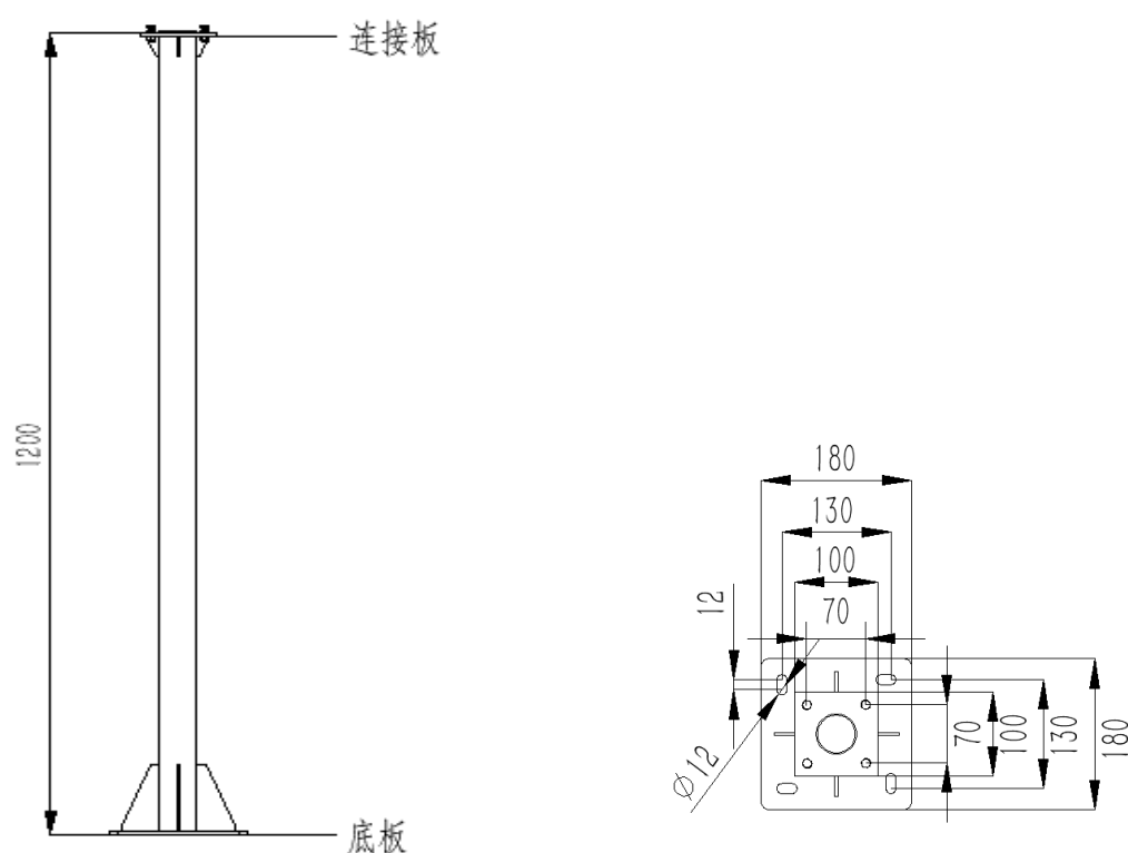
图 1 外形图
