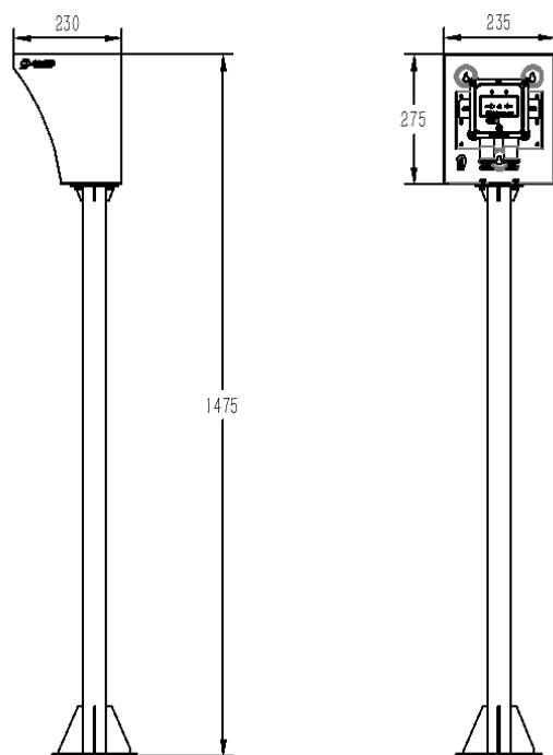
图 2 安装示意图
