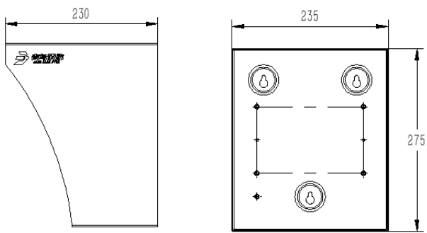
图 1 外形图
