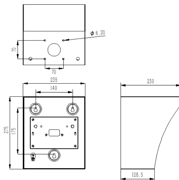
图 2 安装尺寸图
