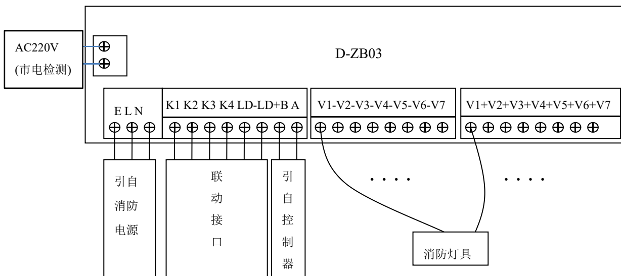
图 3.1 应急照明集中电源接线示意图
